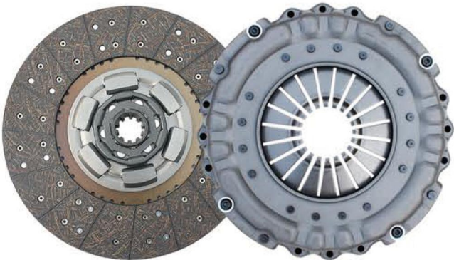
品名：395从动盘总成/压盘总成 Product Name: Pull the 395 driven disc assembly/Cover 规格：395*230*10*44.5/395*230*410 Specification: 395*230*10*44.5/395*230*410 适配车型：东风康明斯 玉柴 Fit models: DFM Cummins Yuchai
