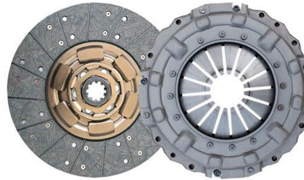
品名：350从动盘总成/压盘总成 Product Name: Pull the 350 driven disc assembly/Cover 规格：350*210*10*38.4/350*210*381 Specification: 350*210*10*38.4/350*210*381 适配车型：玉柴专用 Fit models: YUCHAI
