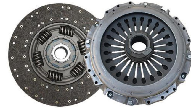
品名: 斯堪尼亚从动盘总成/压盘总成 Product Name: Pull the 430 driven disc assembly/Cover 规格: 430*260*24*52.5/430*240*475 Specification: 430*260*24*52.5/430*240*475 适配车型: 斯堪尼亚 Fit models: SCANIA
