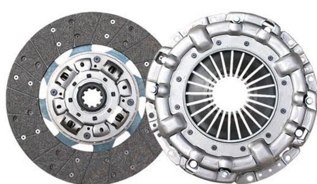
品名: 玉柴325压盘及从动盘总成 Product Name:Yuchai 325 driven disc assembly 规格: 325*190*10*38.1 / 325*200*365 Specification:325*190*10*38.1 / 325*200*365 适配车型: 玉柴 福田 Fit models:Yuchai fukuda
