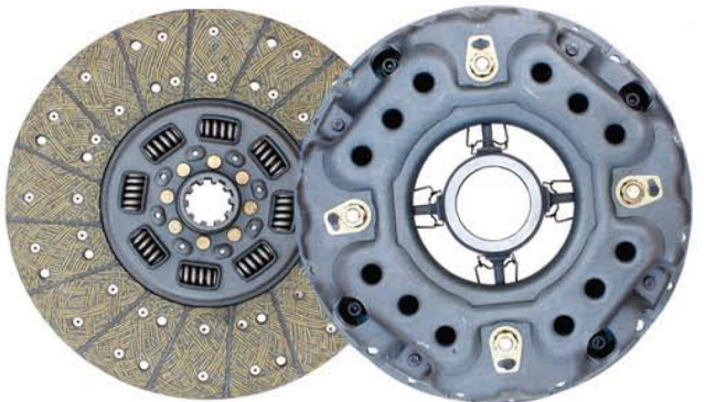
品名：380从动盘总成/压盘总成 Product Name: Pull the 380 driven disc assembly/Cover 规格：380*220*10*44.5/380*200*410 Specification: 380*220*10*44.5/380*200*410 适配车型：东风康明斯 锡柴 柳汽 Fit models: The steam, Liu steam, Cummings, chai
