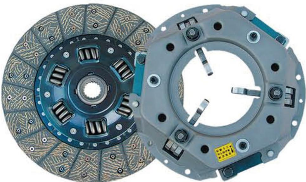
品名: 275TCM压盘及从动盘总成/压盘总成 Product Name: 275 TCM driven disc assembly/Cover 规格: 275*180*18*35/275*180*290 Specification: 275*180*18*35/275*180*290 适配车型: TCM叉车 Fit models: TCM Forklift
