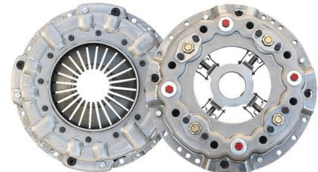
品名: YC350压盘及350CD压盘总成 Product Name:YC350/350CD driven Cover assembly 规格: 352*198*379 / 350*218*379 Specification: 352*198*379 / 350*218*379 适配车型: 玉柴 / 日野 Fit models: Yuchai/Hino
