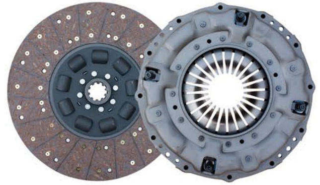
品名: 430九簧从动盘总成/压盘总成 Product Name: Pull the 430 driven disc assembly/Cover 规格: 430*240*10*44.5/430*240*470 Specification: 430*240*10*44.5/430*240*470 适配车型: 一汽解放 福田欧曼 陕汽红岩 玉柴 锡柴 潍柴 Fit models: FAW Yuchai Xichai Weichai Shaanxihongyan
