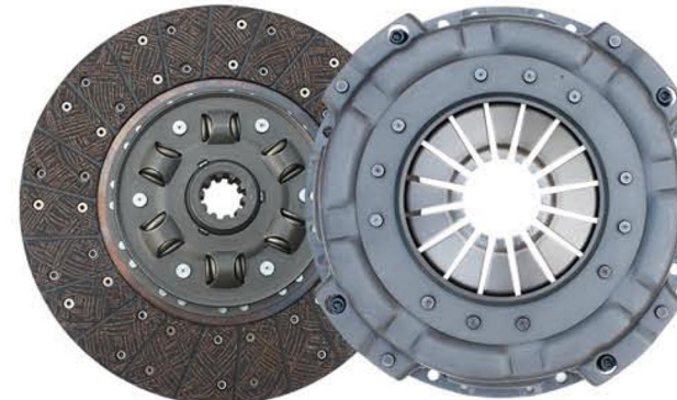
品名：EQ145从动盘总成/压盘总成 Product Name: Pull the EQ145 driven disc assembly 规格：350*210*10*38.4/350*216*381 Specification: 350*210*10*38.4/350*216*381 适配车型：玉柴 东风天锦 Fit models: Dongfeng Tianjin Yu Chai
