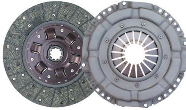
品名: 300从动盘总成/压盘总成 Product Name: Pull the 300 driven disc assembly/Cover 规格: 300*190*350/300*190*10*35 Specification: 300*190*350/300*190*10*35 适配车型: 北汽福田 金龙客车 江淮 解放虎V Fit models: FUKUDA Golden Dragon Bus FAW tiger V
