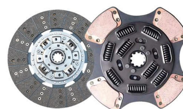
品名: 350解放J6三级减震 /387从动盘总成 Product Name:350 FAW J6 / 387 driven disc assembly/ 规格: 350*210*10*38.4 / 387*10*50.8 Specification:350*210*10*38.4 / 387 *10*50.8 适配车型: 解放J6专用 玉柴/美国拖拖卡车 Fit models:J6 FAW Yuchai American tow truck
