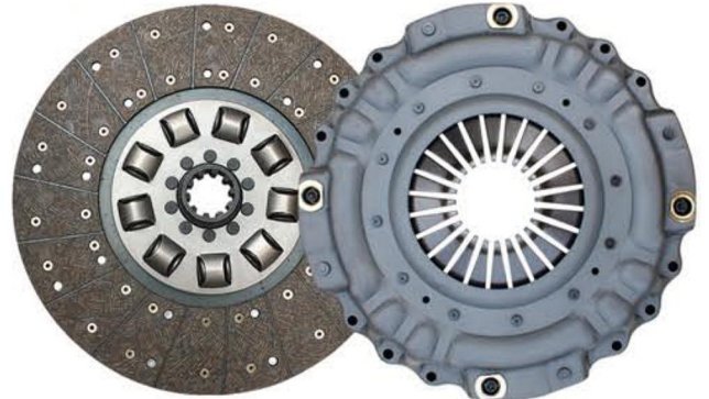
品名: 430从动盘总成/压盘总成 Product Name: Pull the 430 driven disc assembly/Cover 规格: 430*210*10*44.6/430*228*450 Specification: 430*210*10*44.6/430*228*450 适配车型: 东风康明斯 天龙 玉柴 锡柴 潍柴 大金 宇通 Fit models: DFM Cummins Tianlong Yuchai Xichai Weichai Jinlong Yutong
