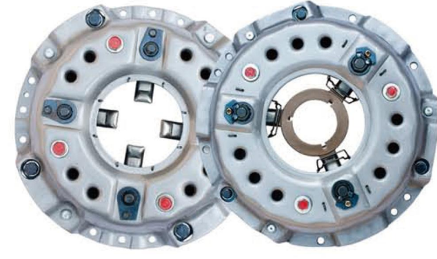
品名: 台励福 / 丰田叉车压盘总成 Product Name:Taiwan Lai Fu/Toyota forklift driven Cover assembly 规格: 275*180*290 Specification:275*180*290 适配车型: 台励福 丰田叉车 Fit models:Taiwan Lai Fu/Toyota forklift
