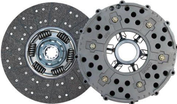
品名：380三级减震从动盘总成/压盘总成/压盘总成 Product Name: Pull the 380 driven disc assembly/Cover 规格：380*220*10*44.5/380*200*410 Specification: 380*220*10*44.5/380*200*410 适配车型：东风康明斯 解放 朝柴 玉柴 Fit models: FMCummins FAW Chaochai Yucha
