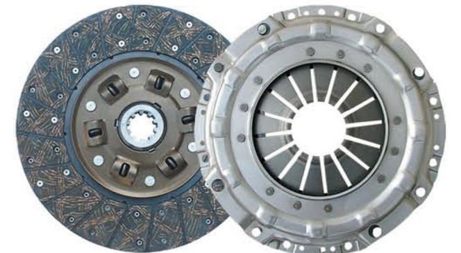
品名：325从动盘总成/压盘总成 Product Name: Pull the 325 driven disc assembly 规格：325*200*10*38.4/325*200*365 Specification: 325*200*10*38.4/325*200*365 适配车型：东风多利卡 江淮 朝柴 大柴 锡柴 Fit models: Dongfeng Duolika JAC Chaochai yuchai xichai
