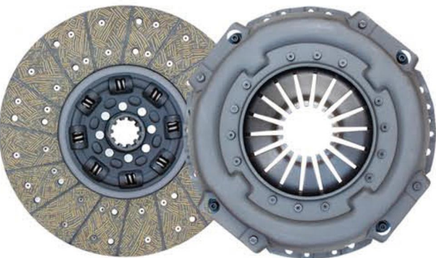
品名：380从动盘总成/压盘总成 Product Name: Pull the 380 driven disc assembly/Cover 规格：380*220*10*44.5/380*200*410 Specification: 380*220*10*44.5/380*200*410 适配车型：东风康明斯 锡柴 柳汽 Fit models: The steam, Liu steam, Cummings, chai
