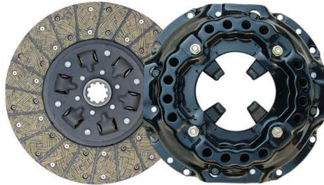
品名: EQ140从动盘总成/压盘总成 Product Name: Pull the EQ140 driven disc assembly/Cover 规格: 325*190*10*38.4/325*190*10*36.5 Specification: 325*190*360/325*190*10*38.4 适配车型: 东风140 扬柴 朝柴 Fit models: DFM140 YANGCHAI CHAOCHAI
