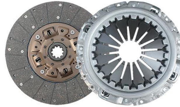
品名: 380欧马可从动盘及压盘总成 Product Name: 380 Aumark driven disc assembly 规格: 380*200*10*44.6/380*216*410 Specification: 380*200*10*44.6/380*216*410 适配车型: 福田 康明斯 欧马可 Fit models: FUKUDA Cummins Oumake
