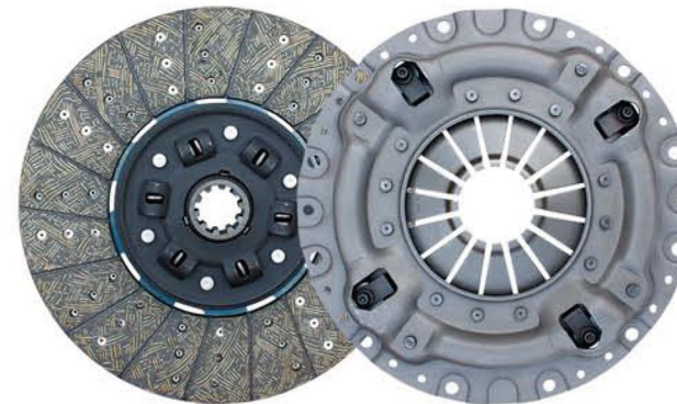
品名：380从动盘总成/压盘总成 Product Name: Pull the 380 driven disc assembly/Cover 规格：380*200*10*44.6/380*200*410 Specification: 380*220*10*44.6/380*210*410 适配车型：一汽解放 Fit models: FAW
