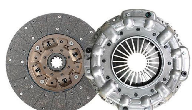
品名: 玉柴380从动盘及压盘及成 Product Name:380Yuchai driven disc assembly/Cover 规格: 380*220*10*44.5 / 380*220*435 Specification:380*220*10*44.5 / 380*220*435 适配车型: 玉柴 福田 Fit models:Yuchai fukuda
