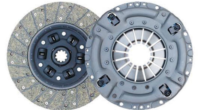
品名：350从动盘总成/压盘总成 Product Name: Pull the 350 driven disc assembly/Cover 规格：350*210*10*38.4/350*210*381 Specification: 350*210*10*38.4/350*210*381 适配车型：解放 锡柴 大柴 Fit models: FAW JIXichai dachai
