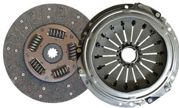
品名: 280压盘及从动盘总成 Product Name:280 driven disc assembly/Cover 规格: 280*180*10*29 Specification:280*180*10*29 适配车型: 依维柯 Fit models:Iveco
