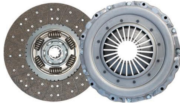
品名：395三级减震从动盘总成/压盘总成 Product Name: Pull the 395 driven disc assembly/Cover 规格：395*230*10*44.5/395*230*410 Specification: 395*230*10*44.5/395*230*410 适配车型：玉柴 解放J6 悍V 龙V 东风天锦 客车 江淮K5 K6L 中卡 Fit models: Yuchai FAWJ6 HanV longV DFMtianjin JAC K5K6
