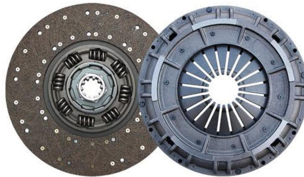
品名: 430三级减震从动盘总成/压盘总成 Product Name: Pull the 430 driven disc assembly/Cover 规格: 430*220*10*50.8/430*225*475 Specification: 430*220*10*50.8 适配车型: 金龙宇通客车 东风天龙雷诺专用 Fit models: Jinlong Yutong Bus DFM Tianlongleiruo
