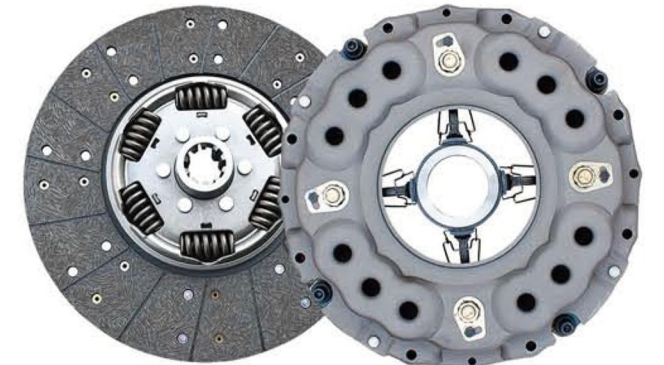
品名：EQ145从动盘总成/压盘总成 Product Name: Pull the EQ145 driven disc assembly 规格：350*210*10*38.4/350*210*381 Specification: 350*210*10*38.4/350*216*381 适配车型：EQ145 玉柴 康明斯 Fit models: EQ145 YUCHAI KANGMINSI
